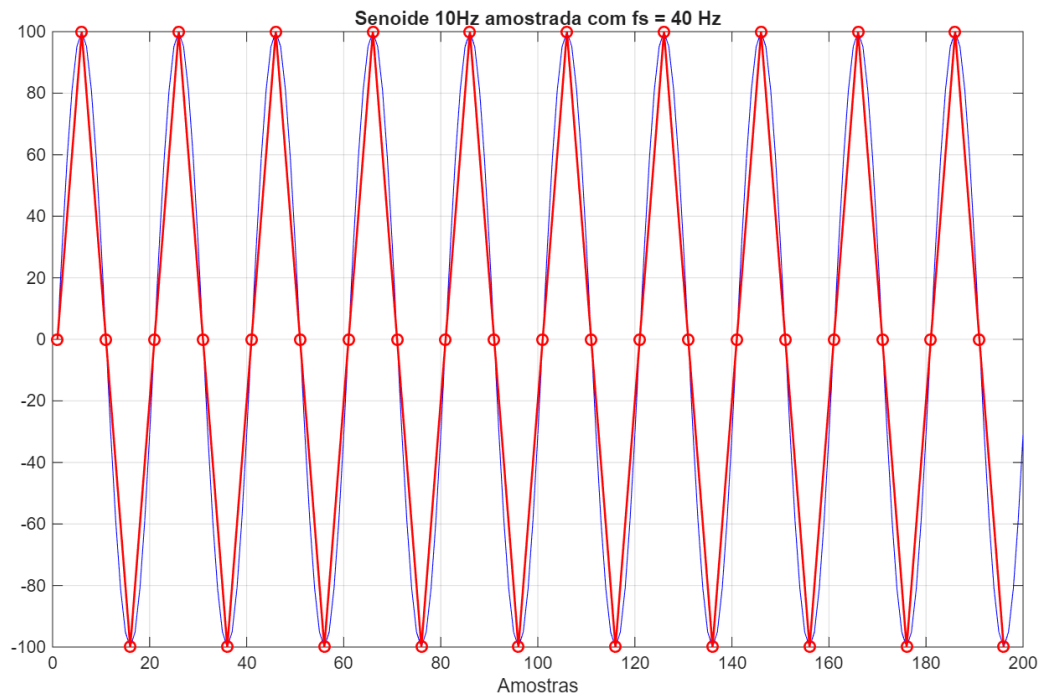
Figura 15: Senoide 10 Hz amostrada a f_s = 40 \text{ Hz} - representação no tempo.
